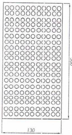
Detail C 2 komada Zaštitna mreža, Polietilen PR144 (podnosiva temp. 125°) - (350x160) \delta = 10 mm
