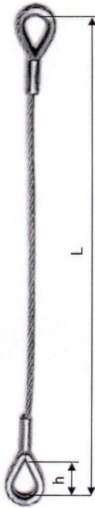
Slika 1. Prikaz jednokrake čelične priveznice omča-omča sa zaštitom (Osiguranje kipera)
