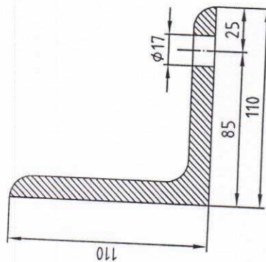
Presjek B-B
