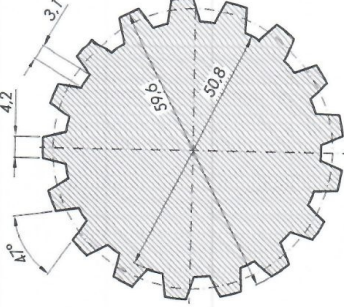
Presjek "B-B"
