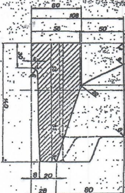
Presjek C-C
